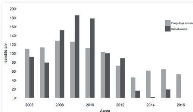
Graafik 14. Ilvese arvukus Eestis 2006–2016 (Allikas: Raido Kont/Tartu ülikooli zooloogia osakond)
