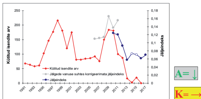
Graafik 13. Ilvese küttimine aastatel 1991–2017 ning ruutloenduse jäljeindeksi muutused. (Allikas: Keskkonnaagentuur)
